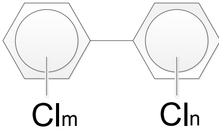
Abb. 1 Allgemeine Strukturformel: C_{12}H_{10-(m+n)}Cl_{m+n}
